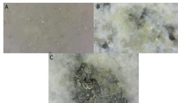
شکل ۷: تصویر میکروسکوپ نوری بعد از ۷ روز تخریب از فیلم: (A) 70%PVA-(B :85%PVA-10%HA-5%ZnO 55%PVA-30%HA-(C و 20%HA-10%ZnO 15%ZnO
