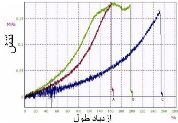
شکل ۵: منحنی تنش/درصد ازدیاد طول، فیلم‌های: (A) 70%PVA-20%HA-(B :85%PVA-10%HA-5%ZnO 55%PVA-30%HA-15%ZnO (C و 10%ZnO
