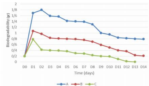
شکل ۶: تخریب‌پذیری بعد از ۱۴ روز، فیلم‌های: (A) 70%PVA-20%HA-(B :85%PVA-10%HA-5%ZnO 55%PVA-30%HA-15%ZnO (C و 10%ZnO
