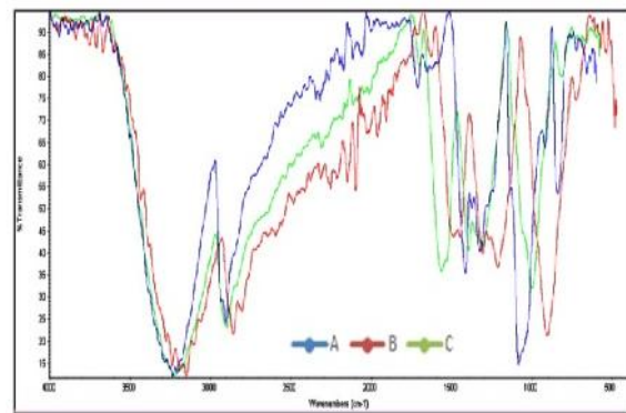
شکل ۵: طیف FTIR از فیلم های: A) 85%PVA-10%HA-5%ZnO (B) 70%PVA-20%HA-10%ZnO (C) و 55%PVA-30%HA-15%ZnO
