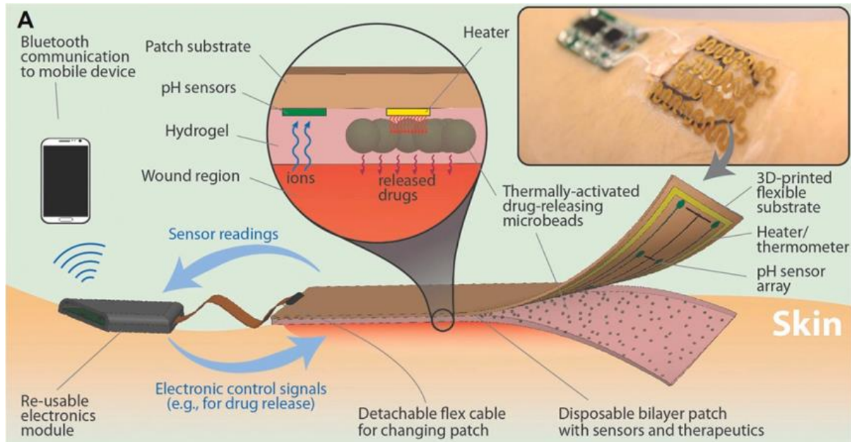
شکل ۳: شماتیک ساختار و نحوه عملکرد زخم‌پوش هوشمند حساس به pH. ۲۱
