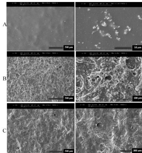
شکل ۳: تصویر میکروسکوپ SEM از فیلم های: (A) 85%PVA-10%HA-5%Zn (B) 70%PVA-20%HA-10%ZnO (C) و 55%PVA-30%HA-15%ZnO
